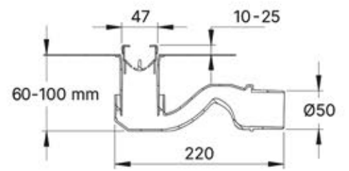
BB-Schnittansicht
