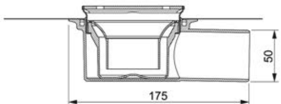
A-A Schnittansicht
