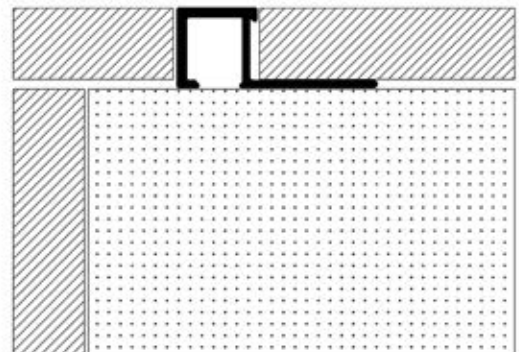
F42 - Abschlussecke
