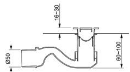
Schnittansicht D-D
